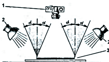
Схема расположения источников света при репродукционной фотосъемке. Цифрами обозначены: 1 — фотокамера; 2 — осветители; 3 — оригинал. Обозначение 2 \alpha показывает угол поля зрения объектива.
